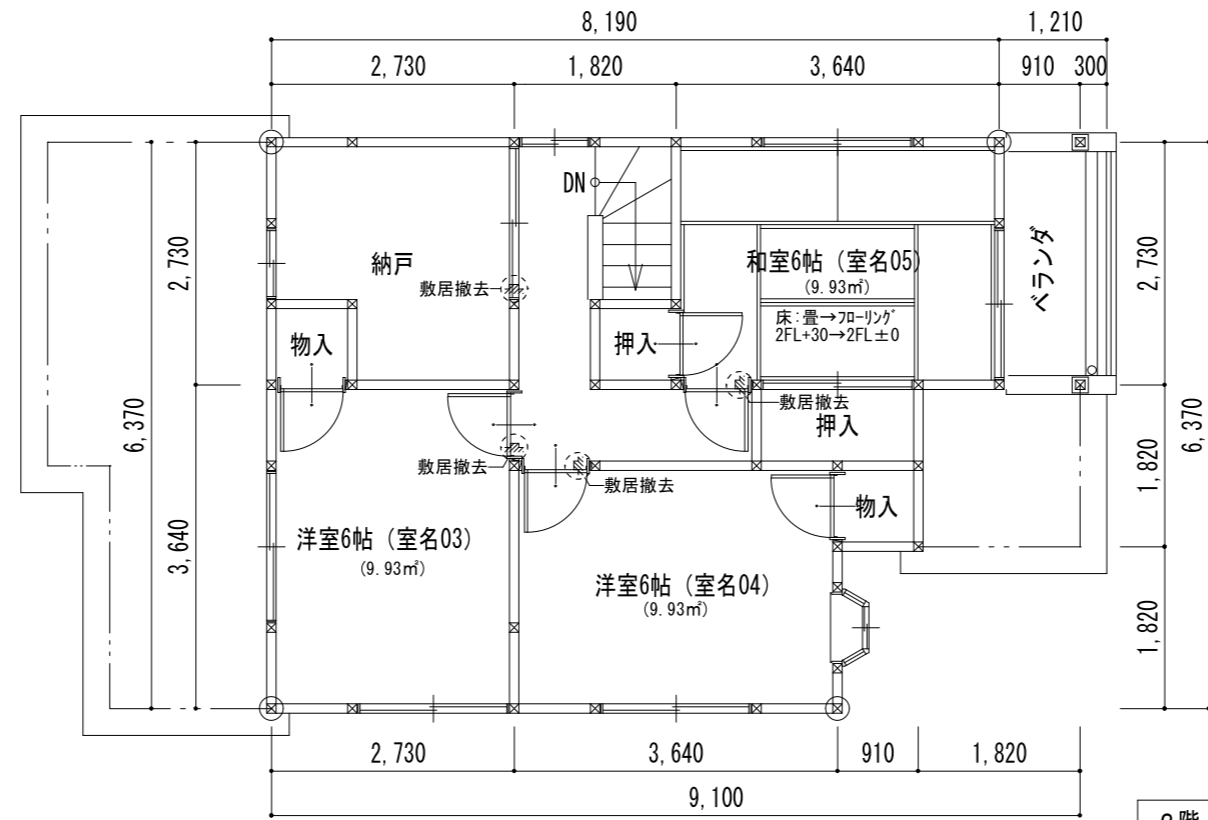
2階 床面積 47.20㎡
